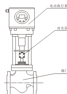
图 3 安装示意
