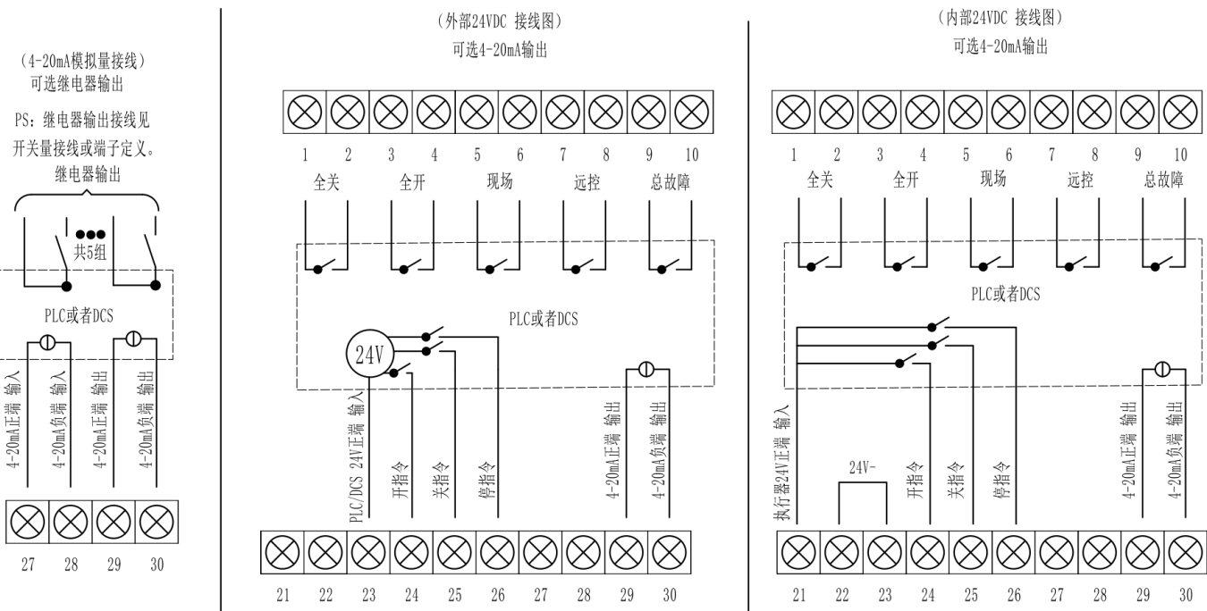
图 6 接线图
