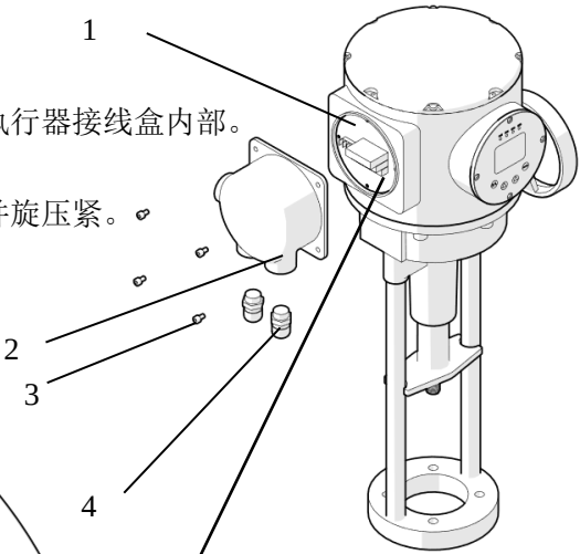
图 4 接线示意图
